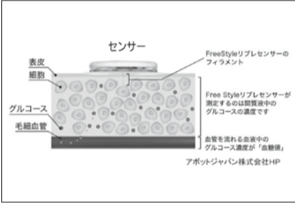
FreeStyleリブレセンサーの仕組み
